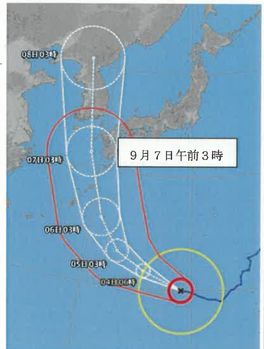
令和2年9月3日6時発表 台風10号進路予想
